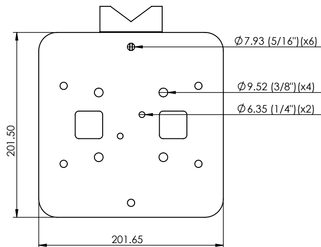
Vista superior
