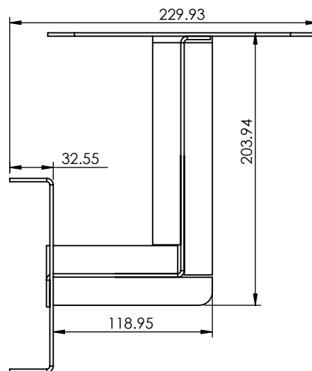
Vista lateral
